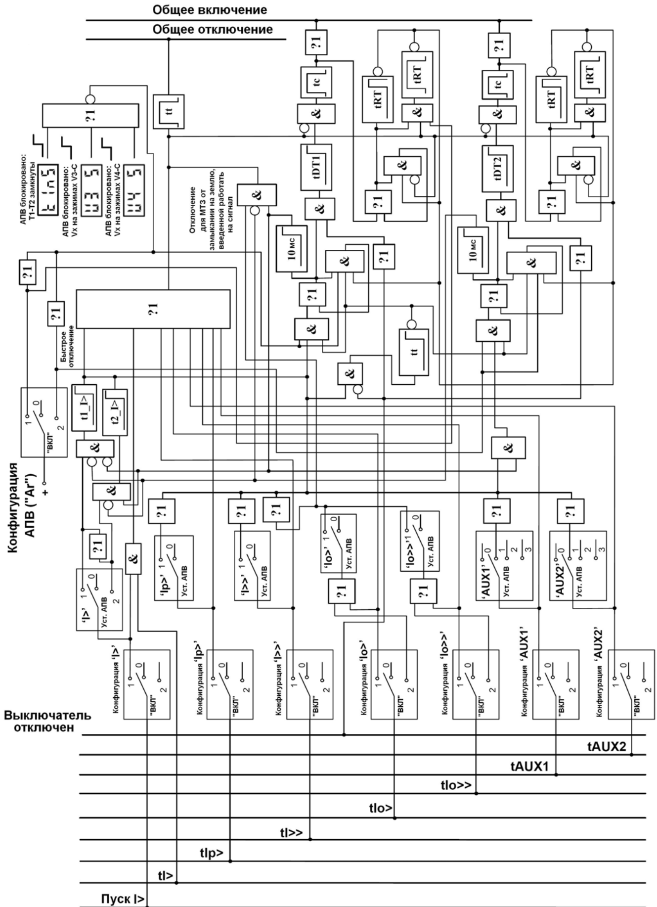
Рис. 13. Логическая схема АПУ
