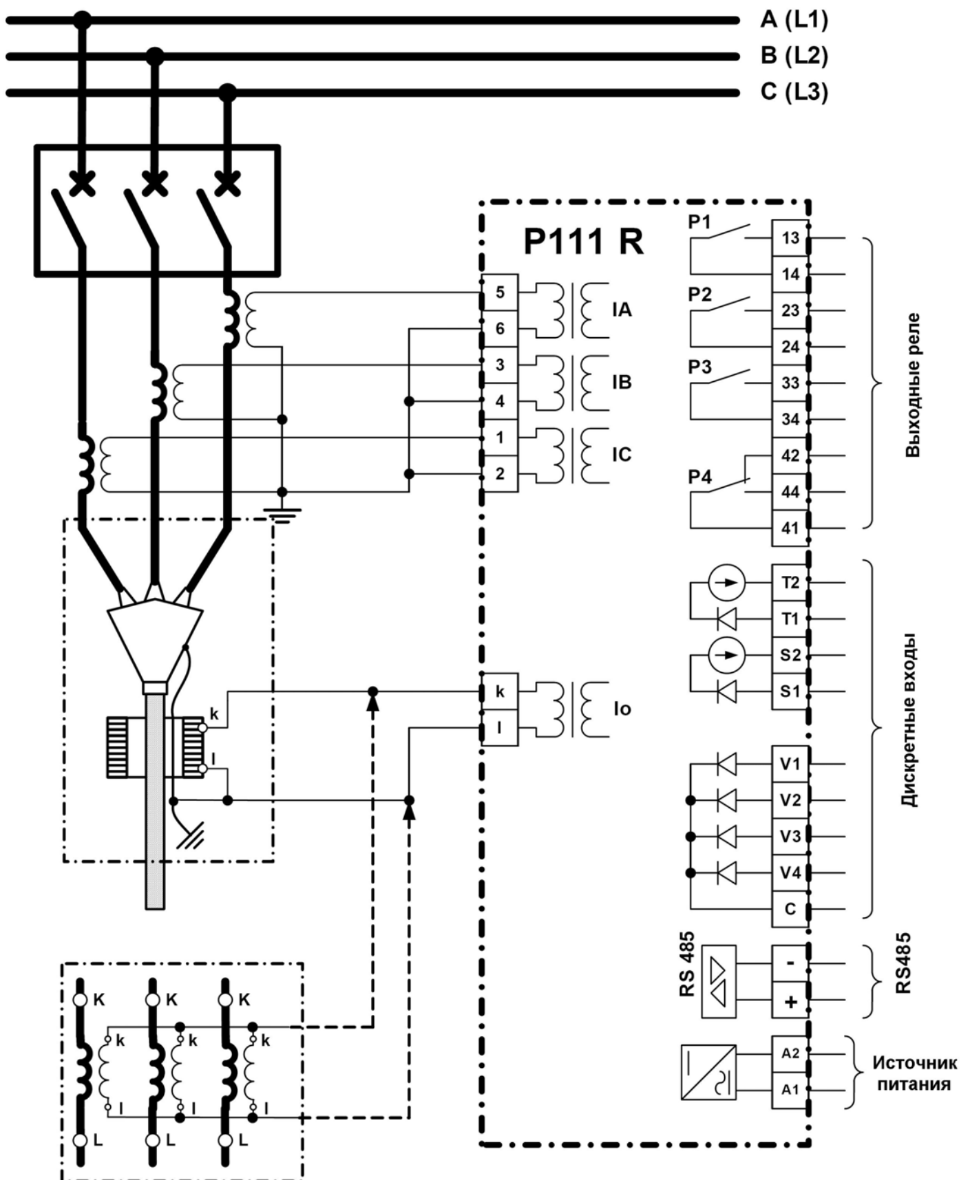
Рис. 19. Схемы подключения
