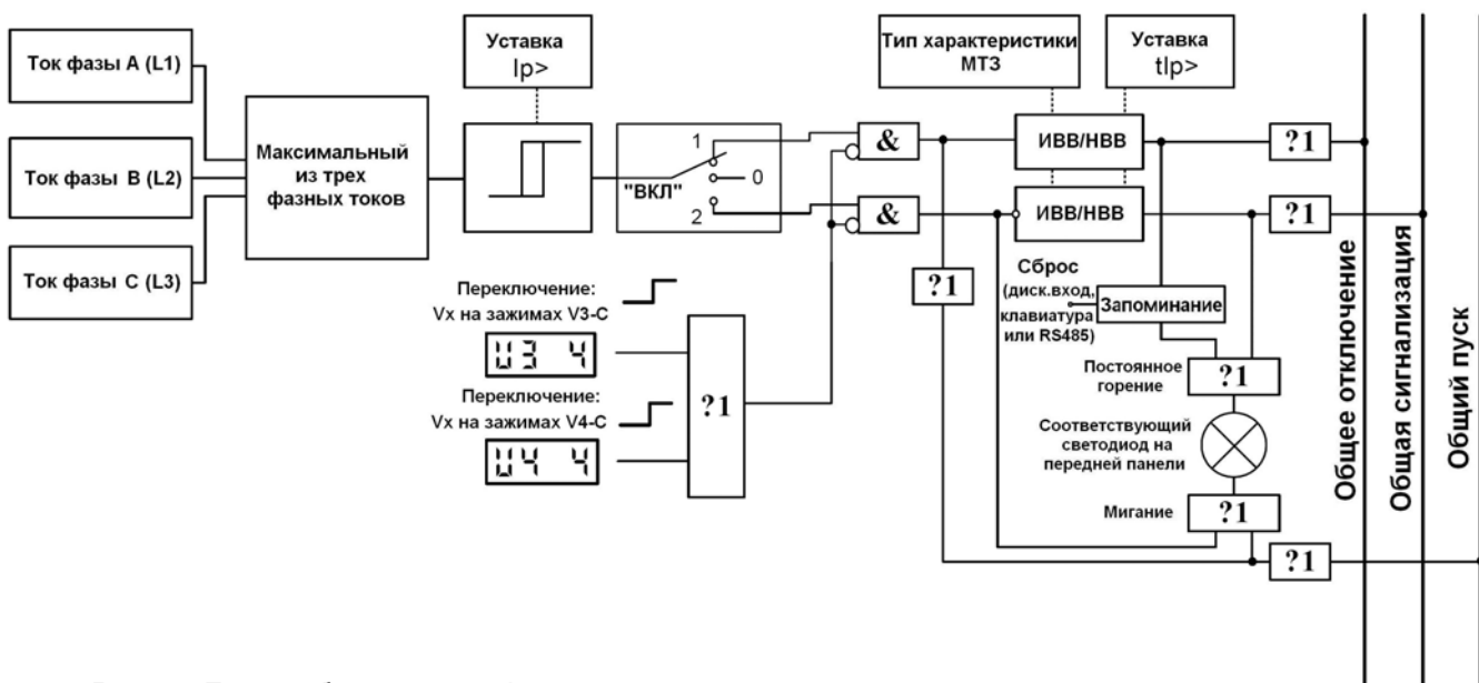
Рис. 7. Логика блокировка tIp>
