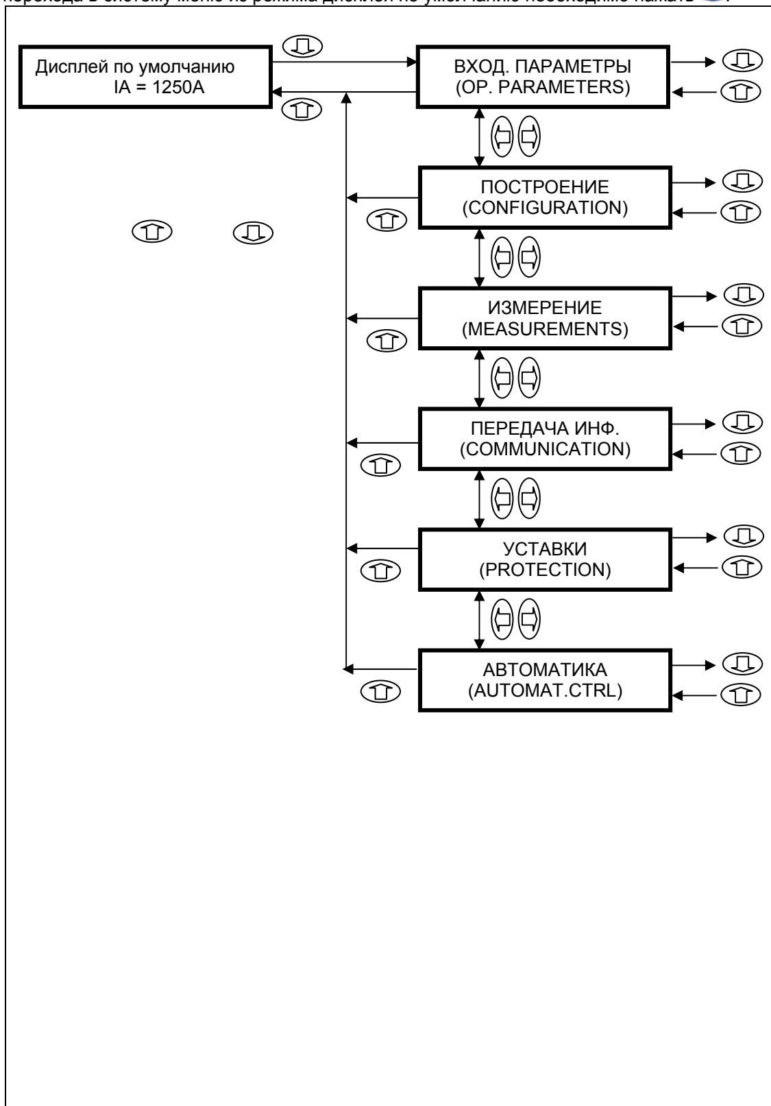
РИС.2 : ОРГАНИЗАЦИЯ ОСНОВНЫХ МЕНЮ MiCOM P120 И P121
