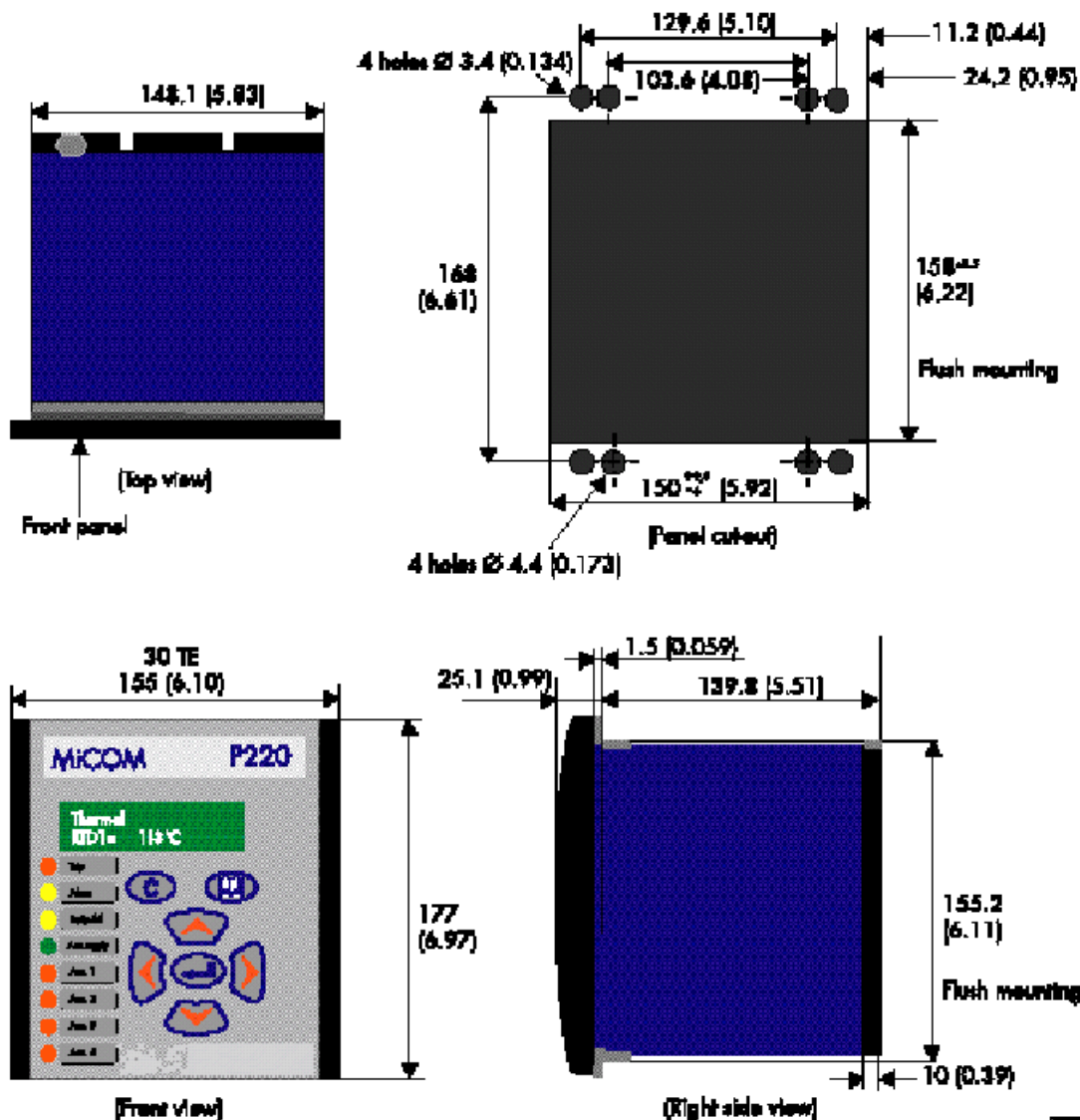
ГАБАРИТНЫЕ РАЗМЕРЫ УСТРОЙСТВ MiCOM P220
