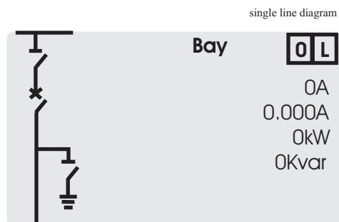
Рисунок 2.20: Однолинейная схема
