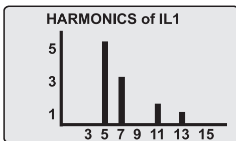
Рисунок 2.12: Пример отображения гистограмм гармоник
