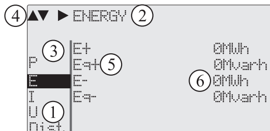
Рисунок 2.2: Секции растрового ЖК-дисплея
