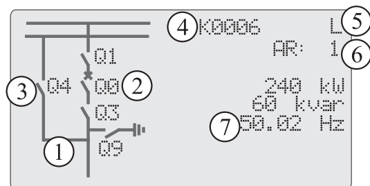
Рисунок 2.1: Секции растрового ЖК-дисплея
