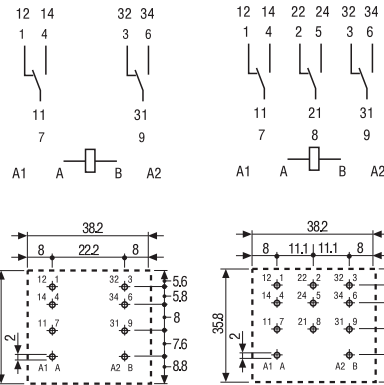
62.22 62.23 Вид со стороны выводов
