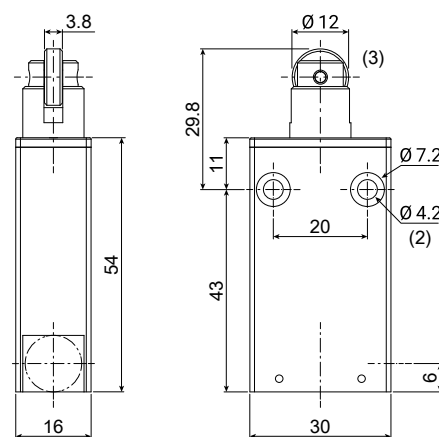
02 roller plunger
