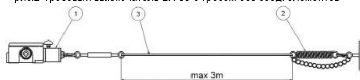
рис.3 Тросовый выключатель LK-30 с тросом с соединительными элементами
