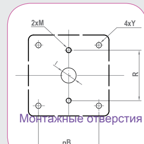
Монтажные отверстия
