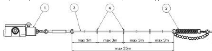
рис.3 Тросовый выключатель LK-30 с тросом с соединительными элементами
