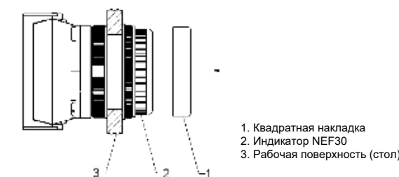
Рис. 2 Установка квадратной накладки на индикаторе NEF30
