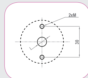
Монтажные отверстия
