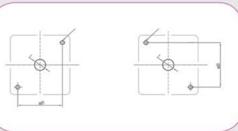
Монтажные отверстия
