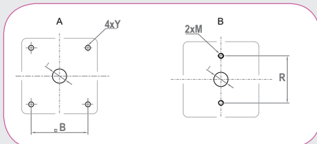
Монтажные отверстия
