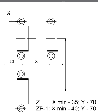
Положение монтажных
