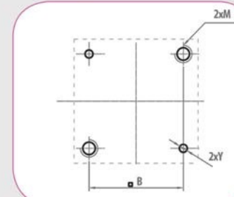
Монтажные отверстия
